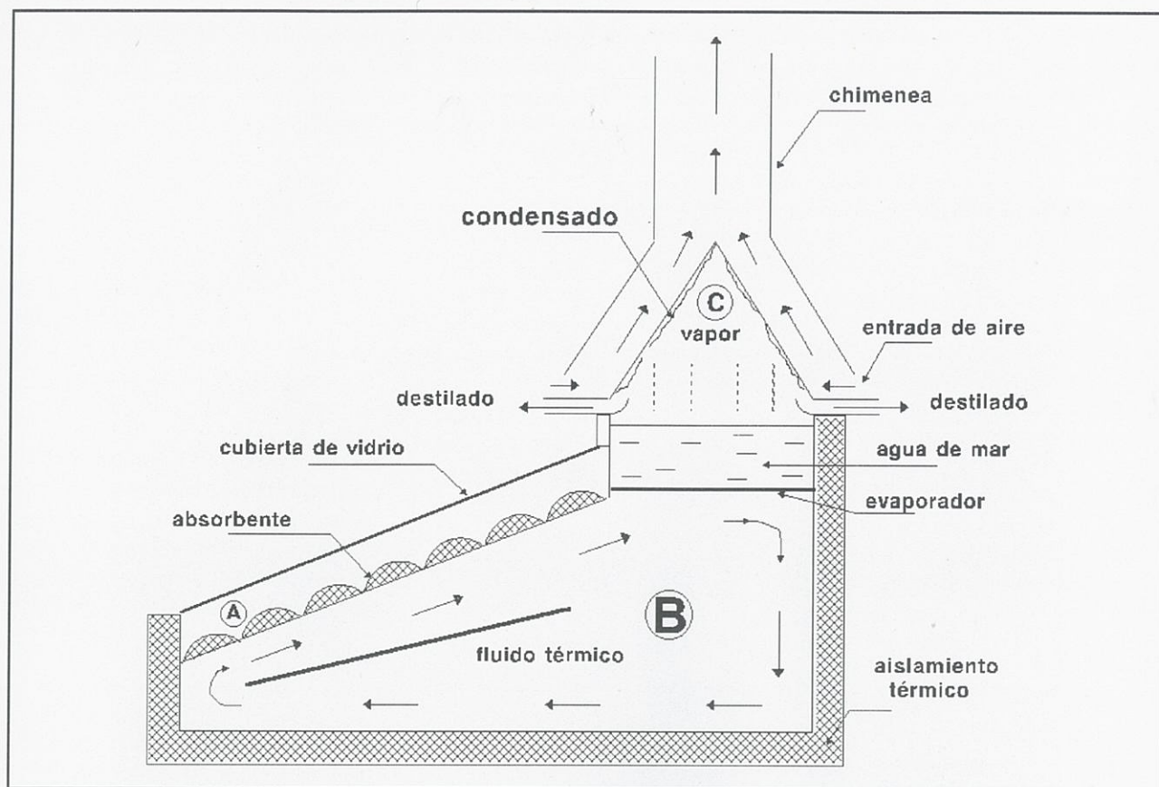
Figura 5. Exemplo d'un diseño de C.D.C. con condensador deseparau.
