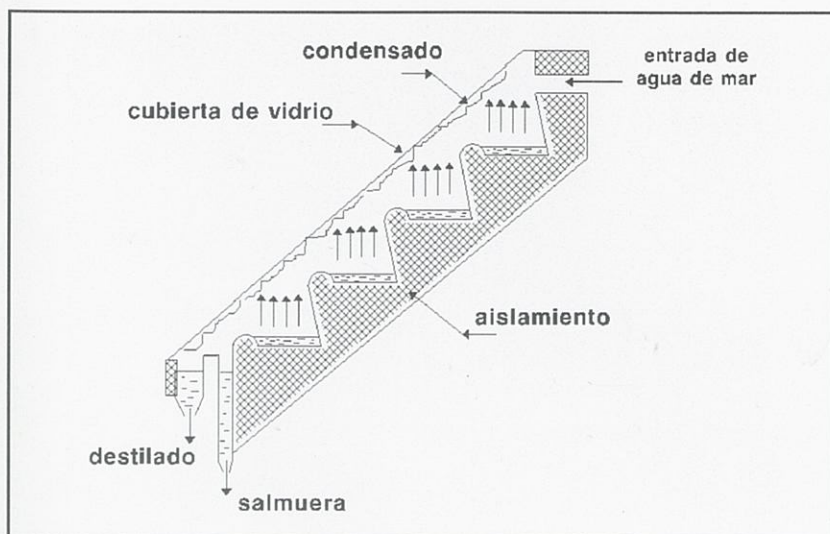
Figura 4. Diseño d'un C.D.C. tipo escalera.
