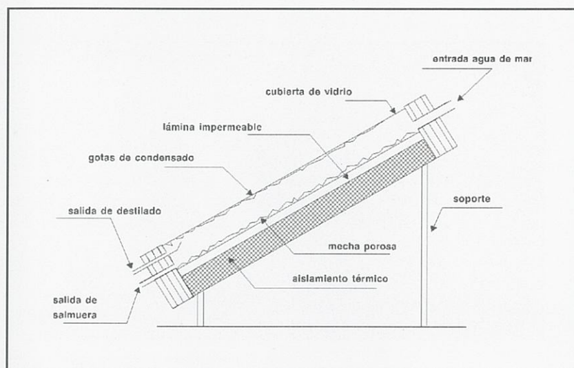
Figura 3. C.D.C. con beta porosa como absorbén.
