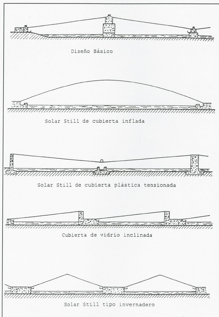
Figura 1. Diferens diseños de Solar Still.
