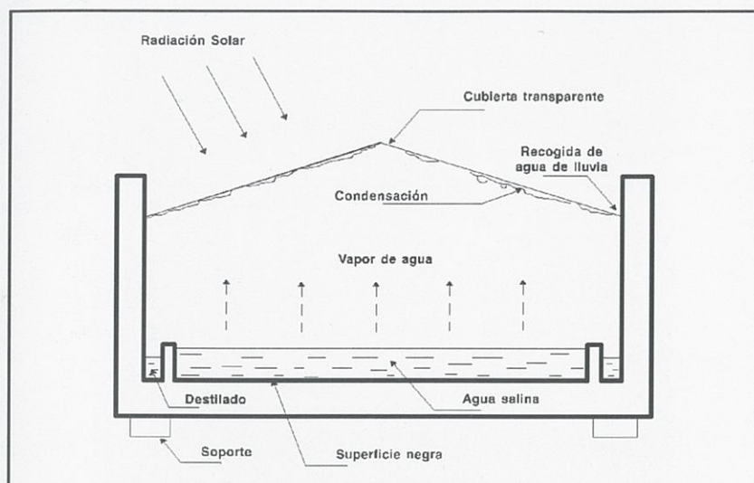
Figura 2. Ejemplo de Aguadere Desaladera Compauta (C.D.C.) típica.
