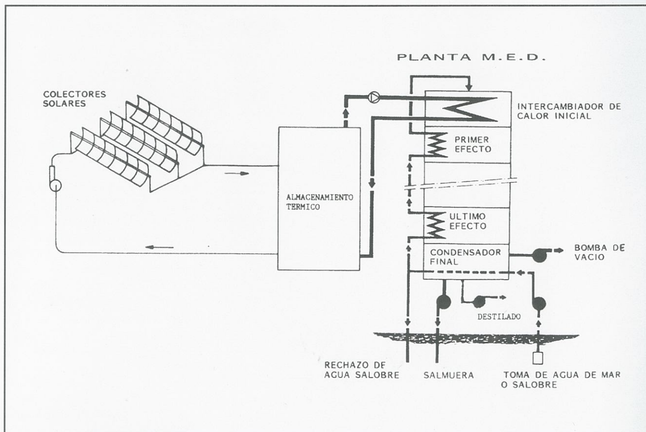
Figura 6. Esquema d'un sistema solar MED típico.
